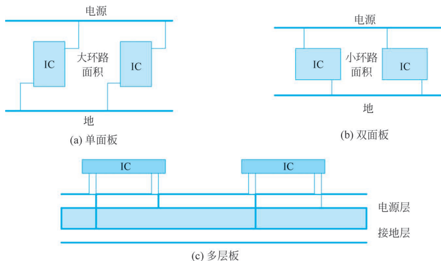
图 5-6 PCB 上的环路面积
