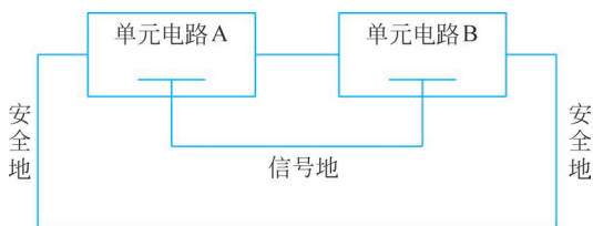
图 5-14 电子系统与设备的浮地
