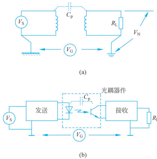
图 5-22 地环路切断
