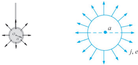
(a) 放在无限大均匀导电媒质中 (b) 放在无限大区域中
