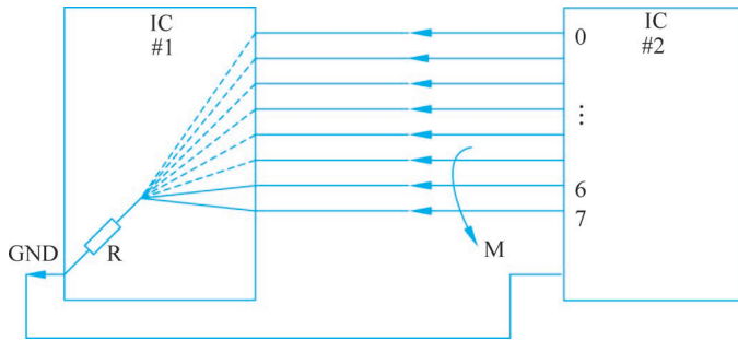
图 5-8 信号环路重叠
