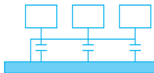
图 5-24 混合接地
