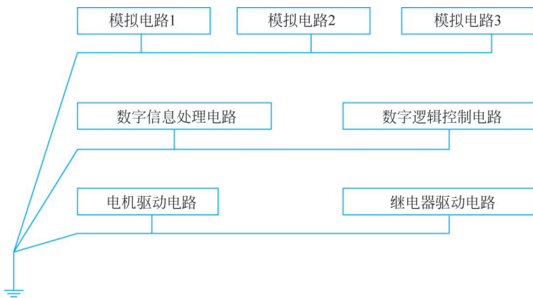
图 5-25 混合接地实例
