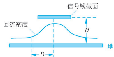
图 5-5 最大信号回流密度
