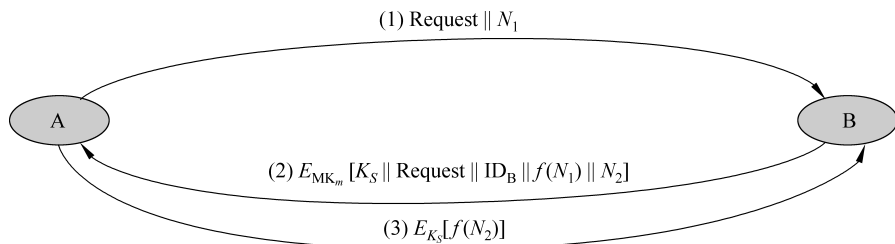
图 5-2 无中心的密钥分配
