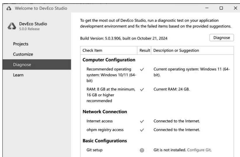
图 1-7 Windows 环境下 DevEco Studio 进入开发环境诊断时的界面
